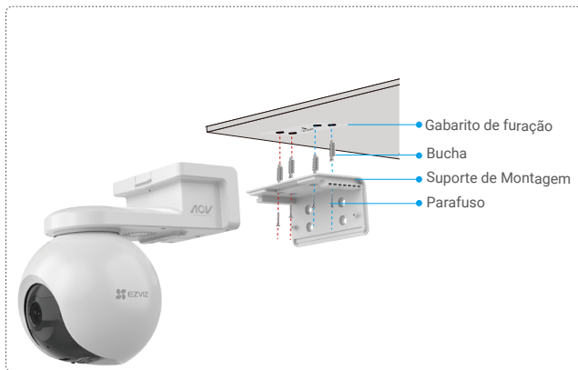
Fig. 1 Montagem no teto
