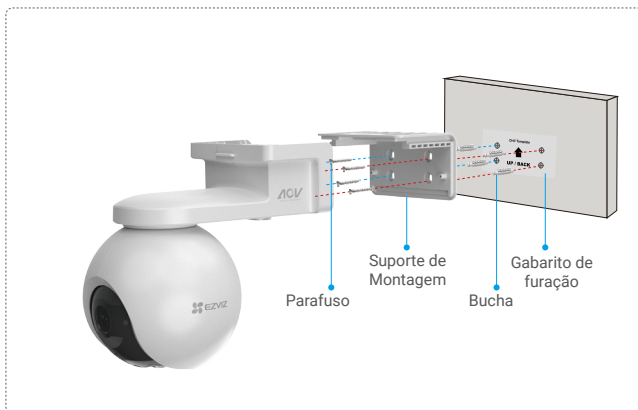
Fig. 2 Montagem na parede
